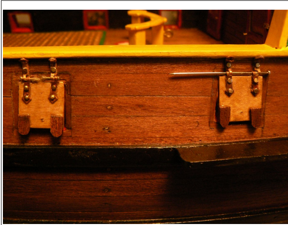
pose des sabords
